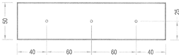
Pamje Siper
