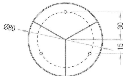
Pamje Siper
