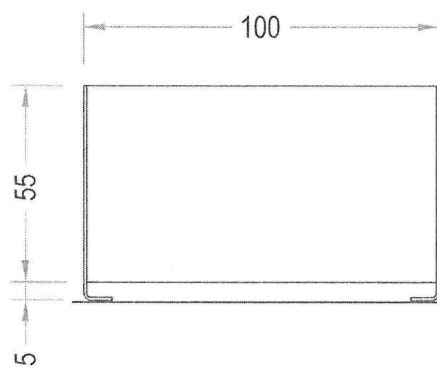
Pamje Siper
