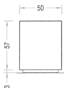
Pamje Anesore
