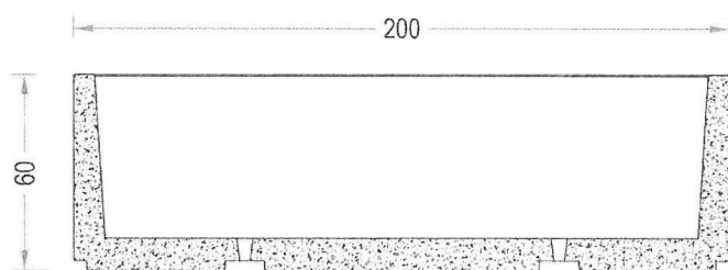
Prerje Gjatesore
