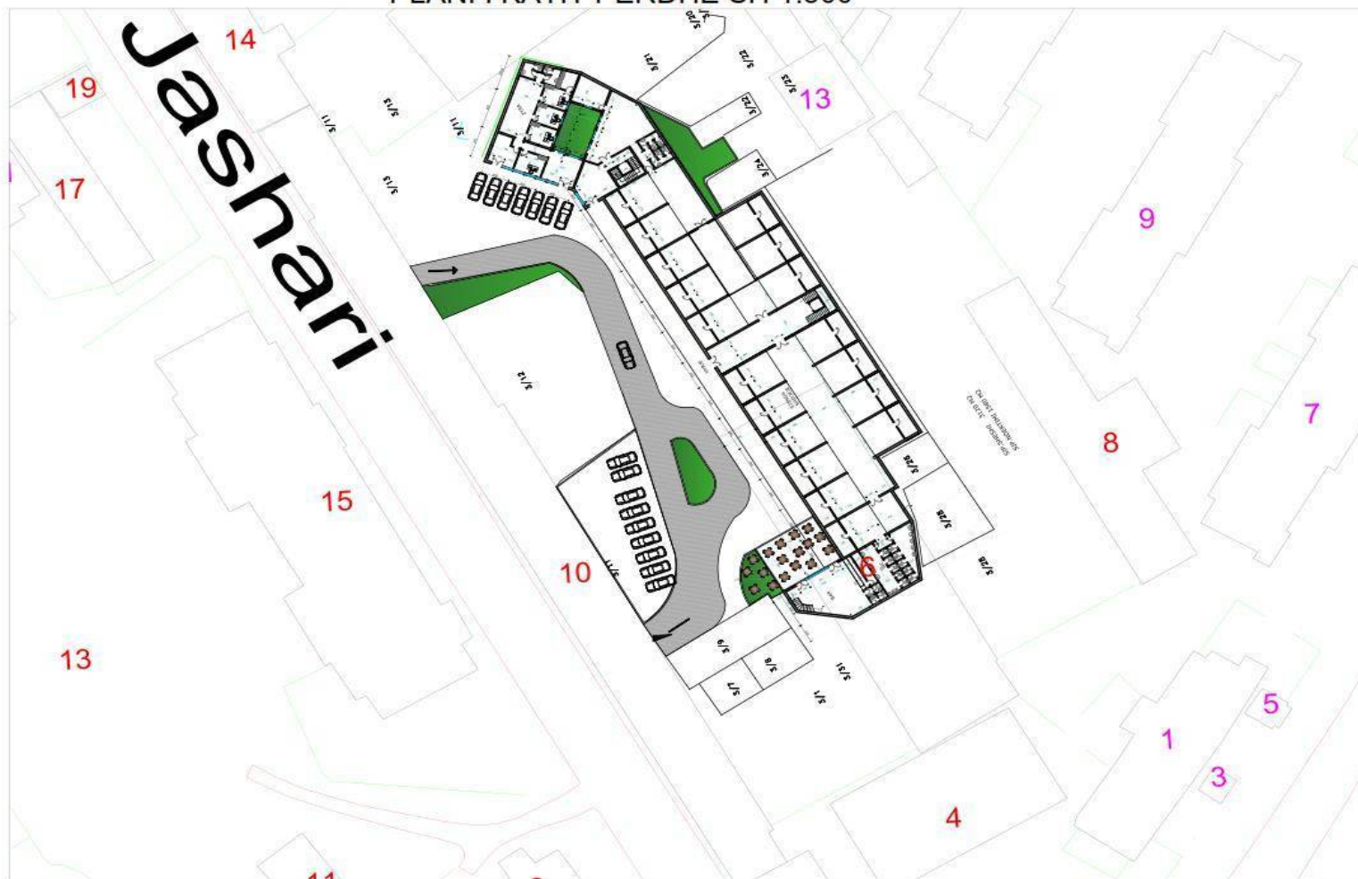
TREGU TEK PARKU I AUTOBUSAVE PLANI I KATIT PERDHE SH 1:500
