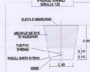
PRERJE KANALI SHKALLA 1:25
