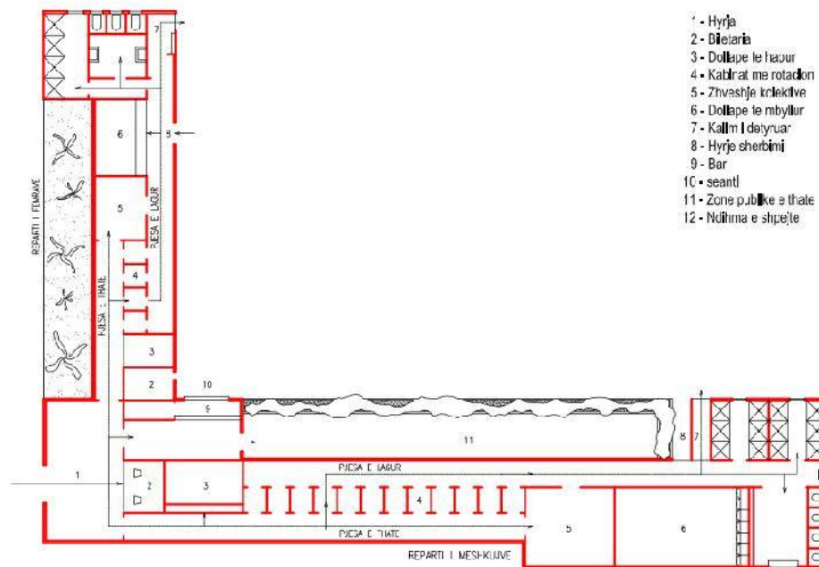
PLANIMETRIA E DHOMAVE TE ZHVESHJEVE TE PISHINAVE Sh 1:150
