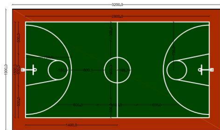
Prerje gjatësore
