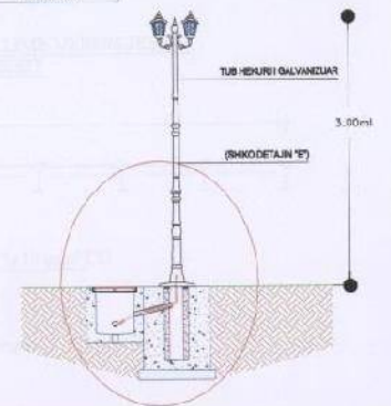
SHITJE E TINGATIT SHKALLA 1:50
